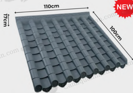
TẤM 100*110 XANH GHI
