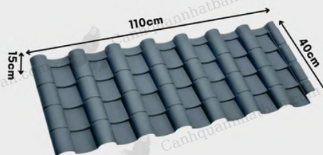
TẤM 40*110 (B) XANH GHI
