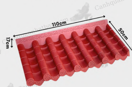
TẤM 50*110 ĐỎ ĐỎ
